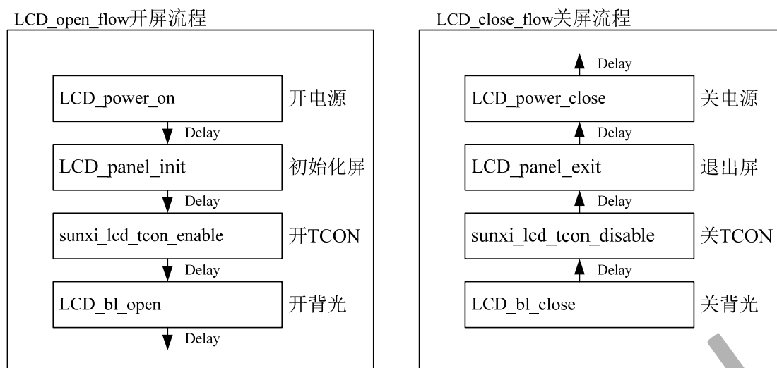
图 6-1 开关屏流程
