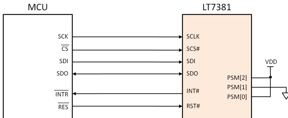
图 2-7: MCU 4 线 SPI 串联接口电路图
