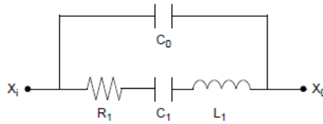
图 A-4: 晶振等效电路图
