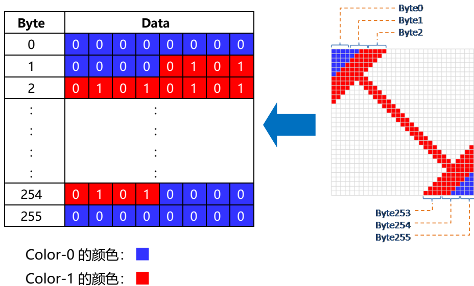
图 8-11: 图形光标范例
