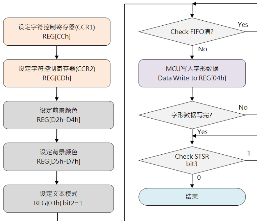
图 8-1: 使用内建字库流程图
