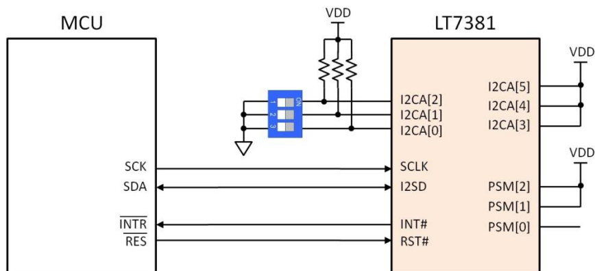
图 2-10: MCU I2C 串联接口电路图
