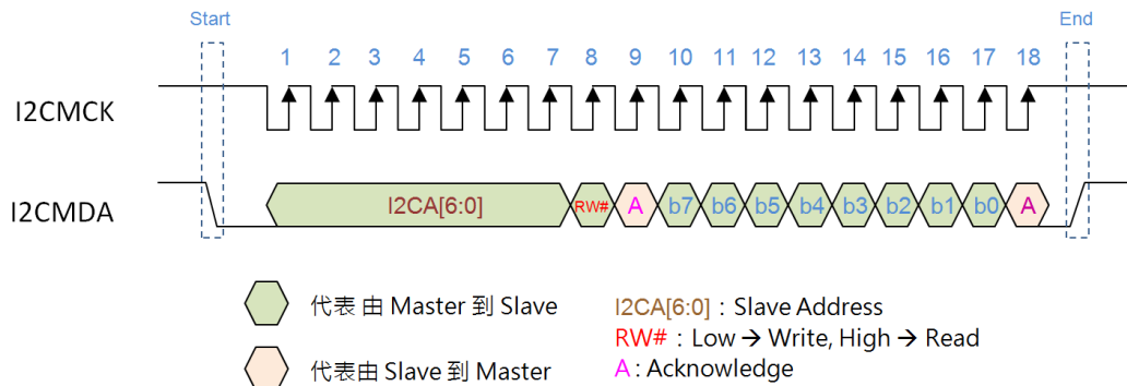
图 10-2: I2C 通讯协议
