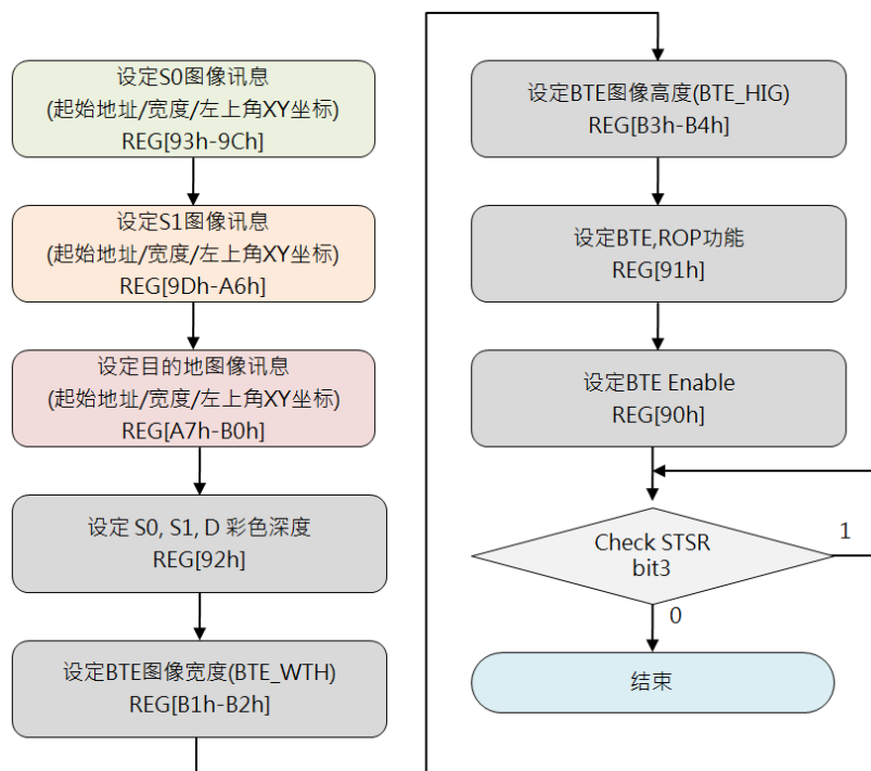
图 7-7: 结合光栅操作的 BTE 内存复制流程图(1)
