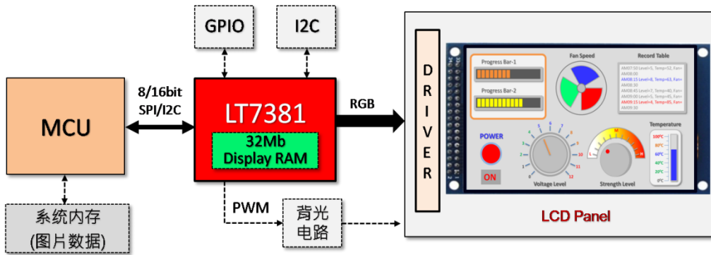
图 A-2: LT7381 系统方块图
