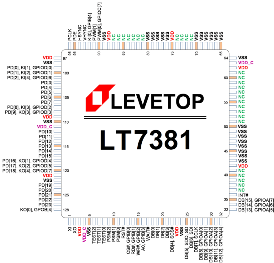
图 A-3: LT7381 引脚图 (LQFP-128Pin)
