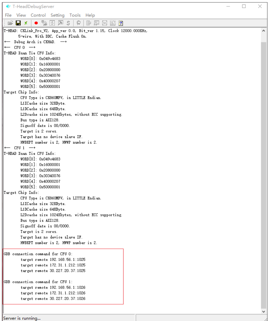
图 8-17 UI 版本 DebugServer 已多核多单端口连接 CK860MP 显示
