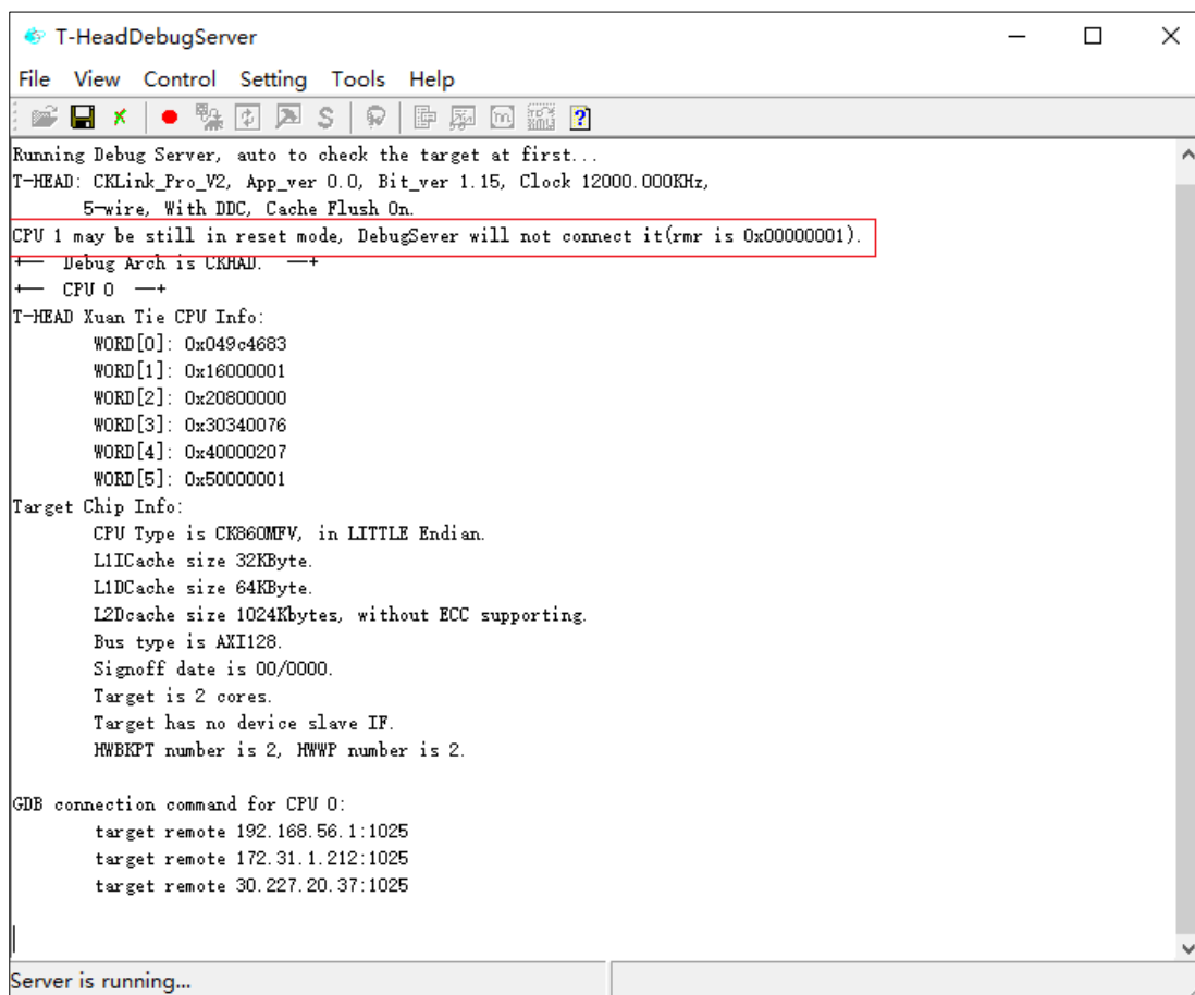
图 8-3 UI 版本 DebugServer 首次连接刚上电的 CK860MP
