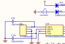
电池电路
