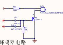
蜂鸣器电路
