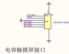
电容触摸屏接口
