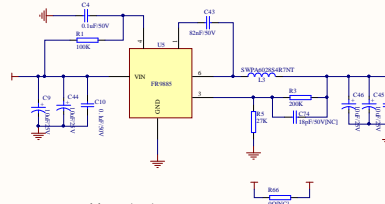
12V转5V电路
