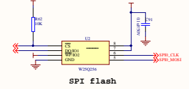
SPI flash
