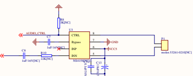
音频电路
