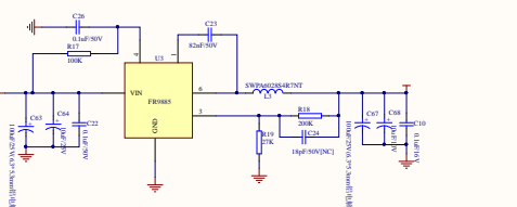
12V转5V电路
