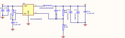
系统3.3V供电
