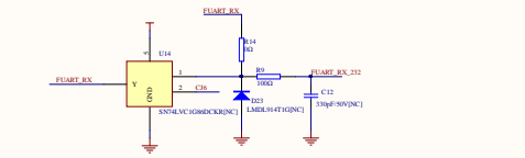
RS232/TTL转换电路
