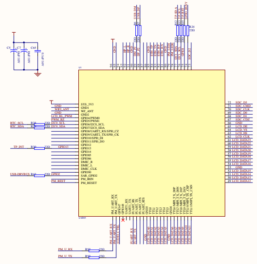
ID0-SOM2D01-V1 核心板
