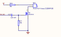
蜂鸣器电路
