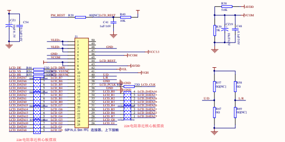
7寸TN92接口
