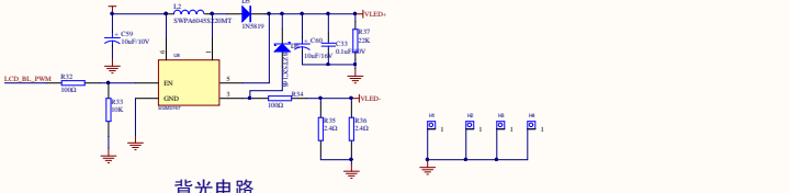
背光电路
