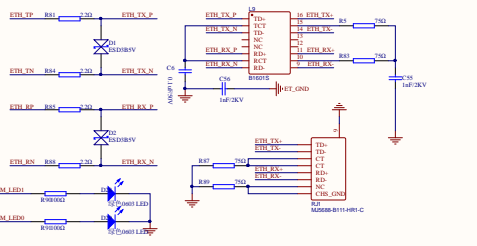
以太网接口
