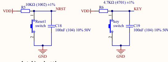
复位电路
