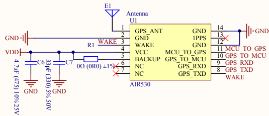
GPS模块
