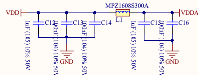
电源电路
