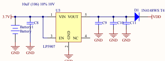
电源电路
