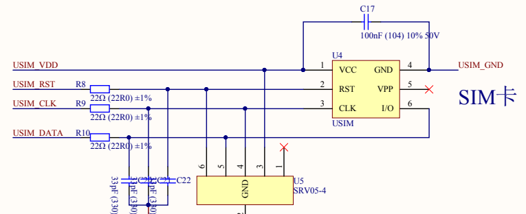
静电保护
