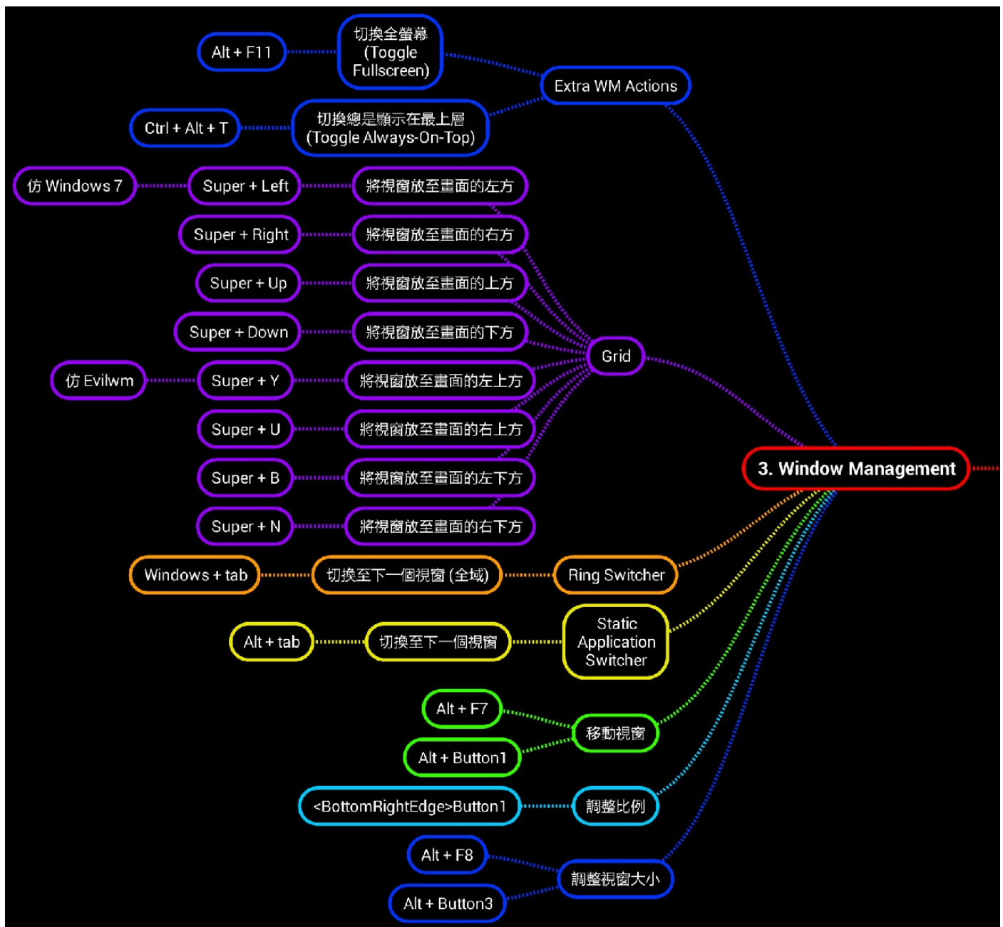
▲ 圖 6: Window Management 分類的設定。
