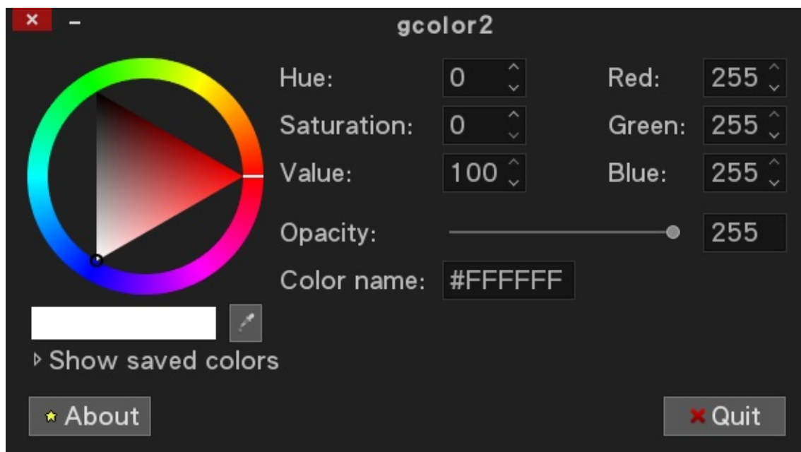
▲ gcolor2 截圖。
